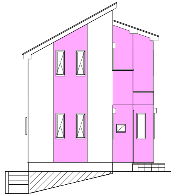
西側 立面図 S:1/100
