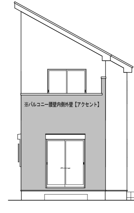
南側 立面図 S:1/100
