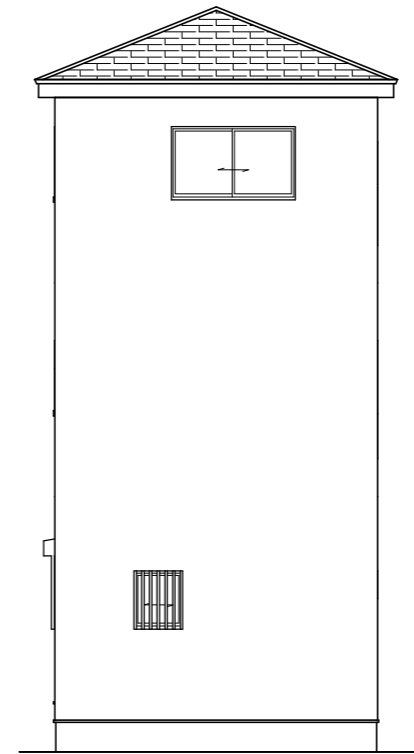
東側 立面図 S:1/100
