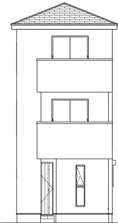
東側 立面図 S:1/100
