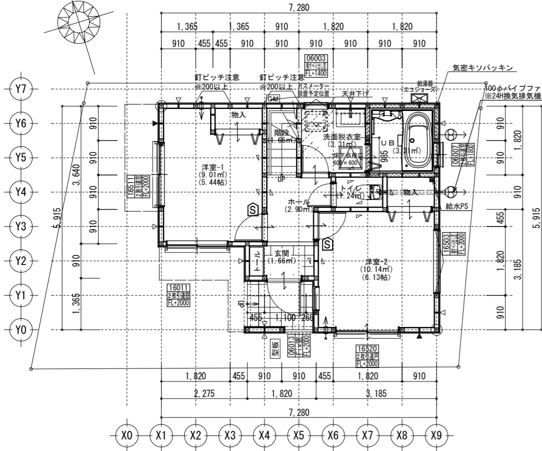
1階 平面詳細図 S:1/100
