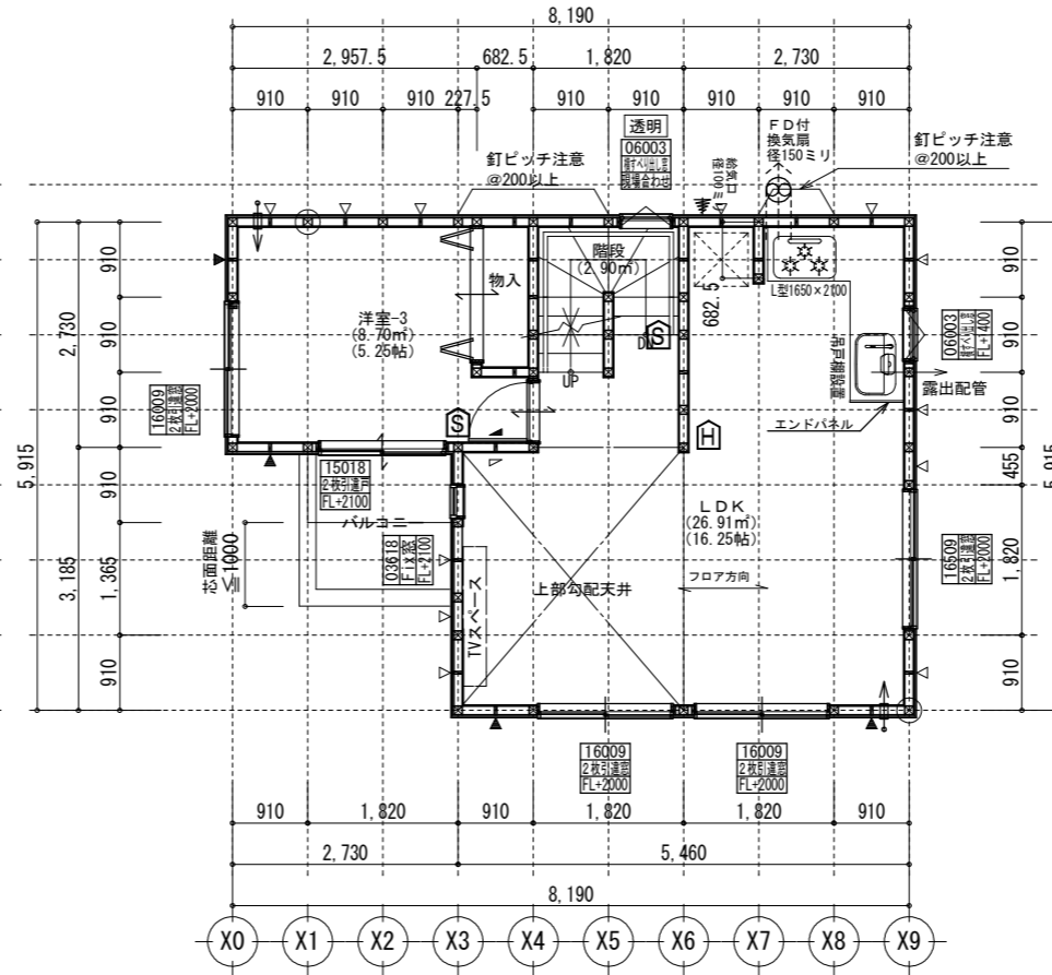
2階 平面詳細図 S:1/100
