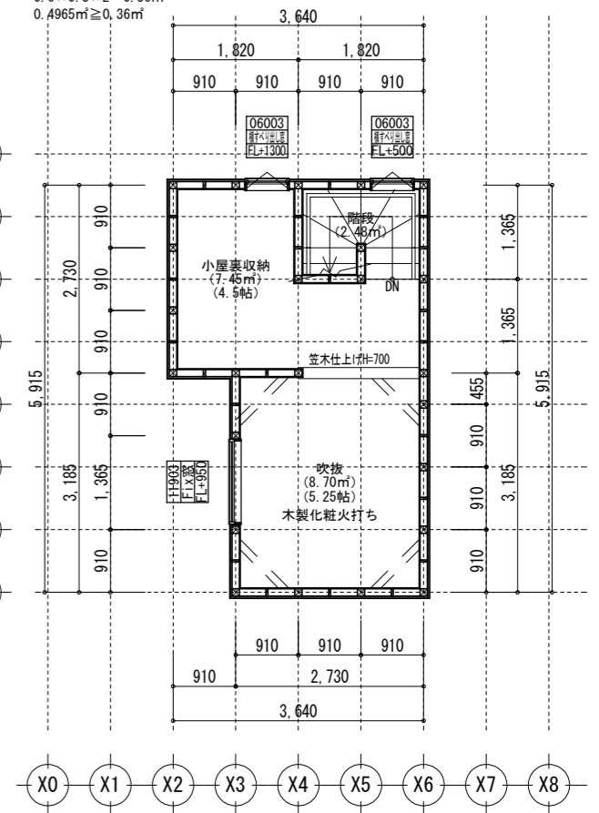
R階 平面詳細図 S:1/100
