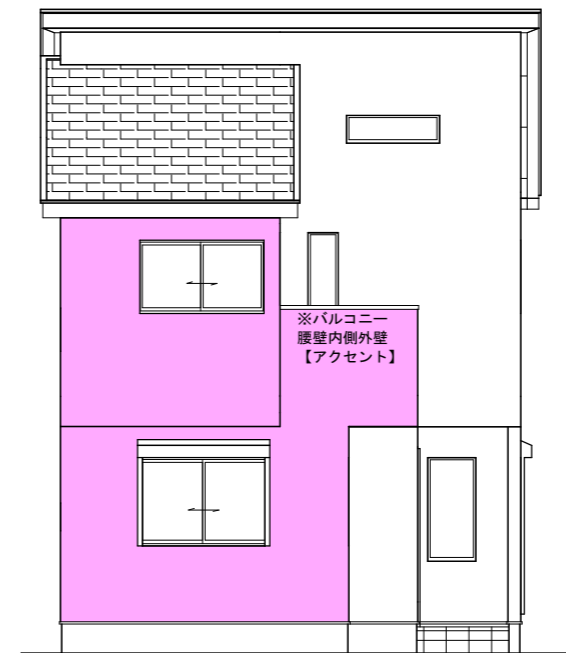
西側 立面図 S:1/100
