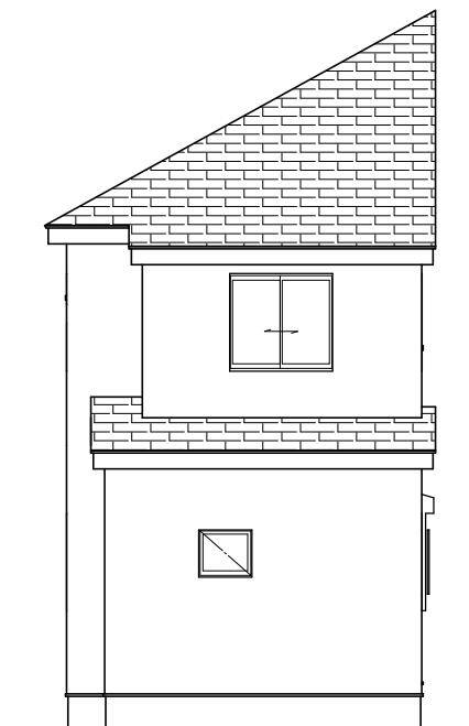
北側 立面図 S:1/100
