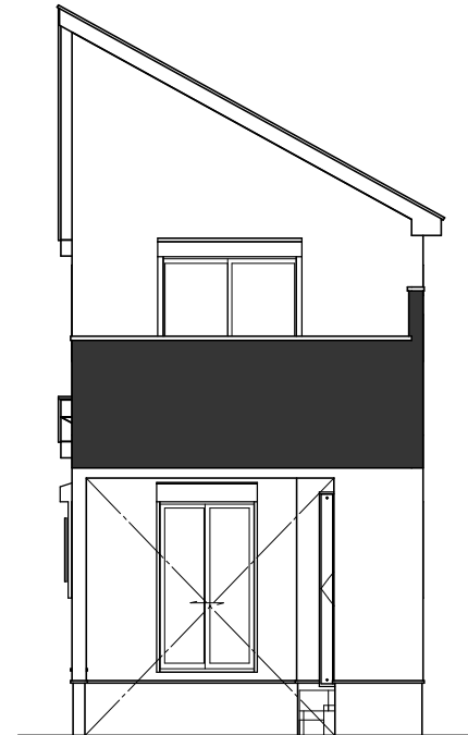
南側 立面図 S:1/100
