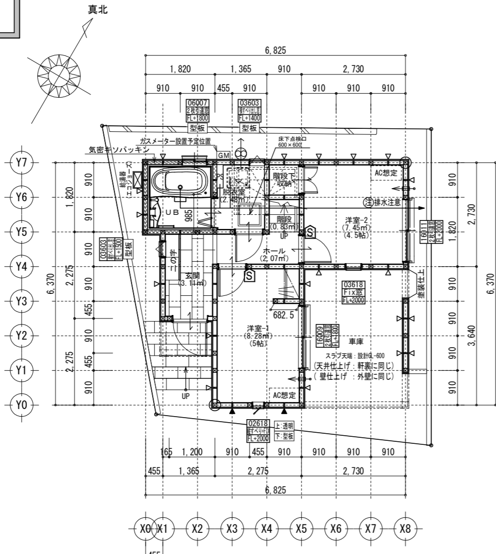
1階 平面詳細図 S:1/100
