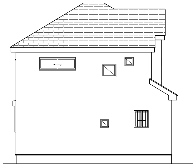
北側 立面図 S:1/100
