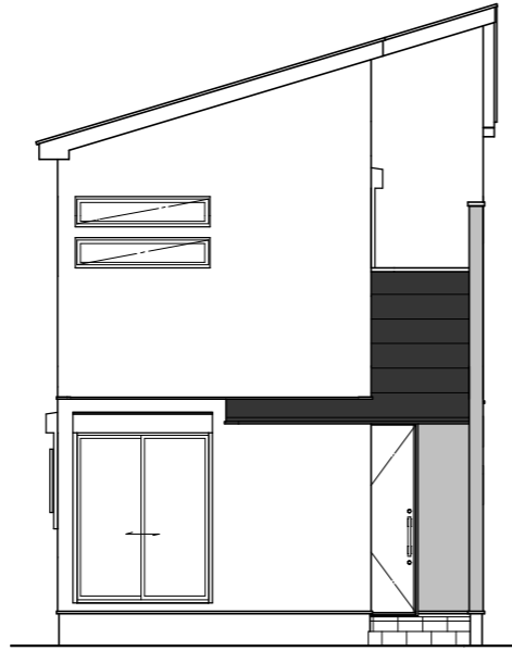
南側 立面図 S:1/100
