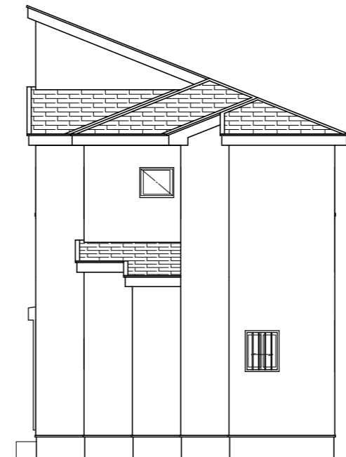
東側 立面図 S:1/100
