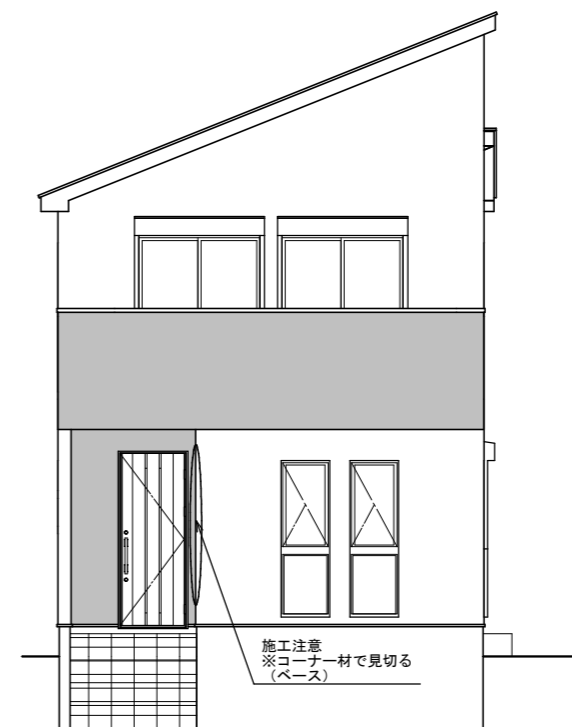
西側 立面図 S:1/100
