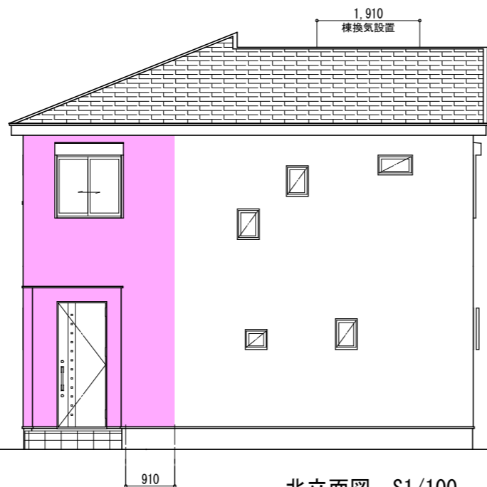
北立面図 S1/100
